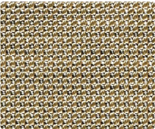
Pyrite 4051-02
